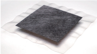
PEM水電解装置用膜電極接合体 (MEA) Membrane Electrode Assemblies (MEA) for PEM electrolyzers
