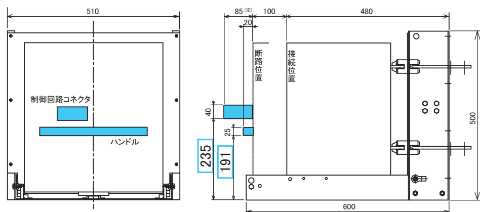
第 46 図 VHB-6J13S(VHB-6H8S,VHB-6J20S,VHB-6J20S-T25)の引出装置収納状態
