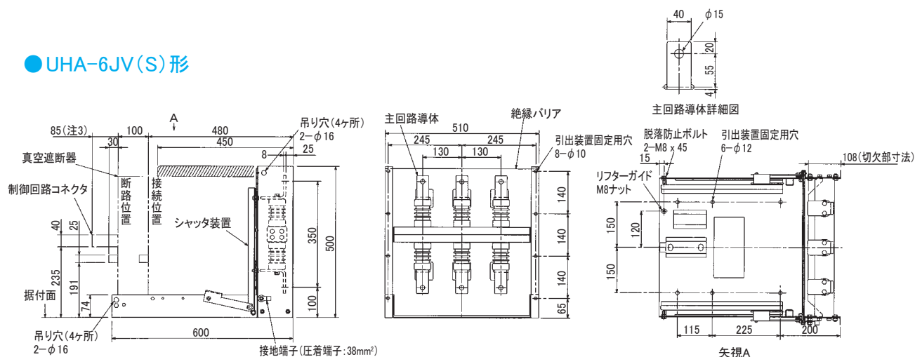
第 18 図 UHA-6JV(S)形引出装置外形寸法図
