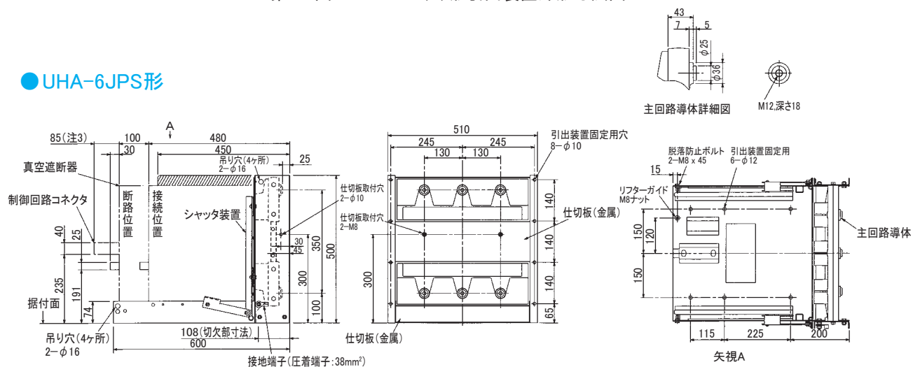
第 19 図 UHA-6JPS形引出装置外形寸法図
