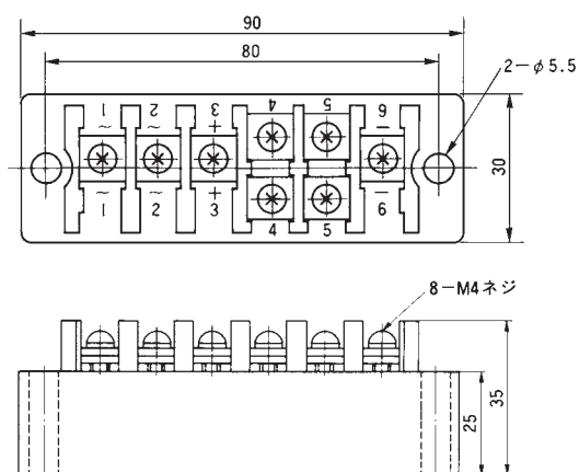
(外形寸法図)
