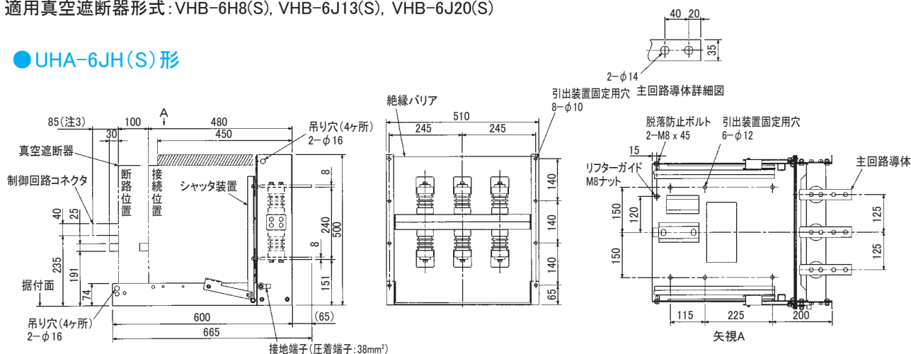
第 17 図 UHA-6JH(S)形引出装置外形寸法図
