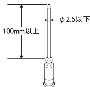
第28図 推奨油差し
