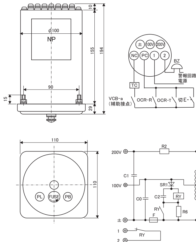
第30図 コンデンサ引外し装置CIT-10Q
