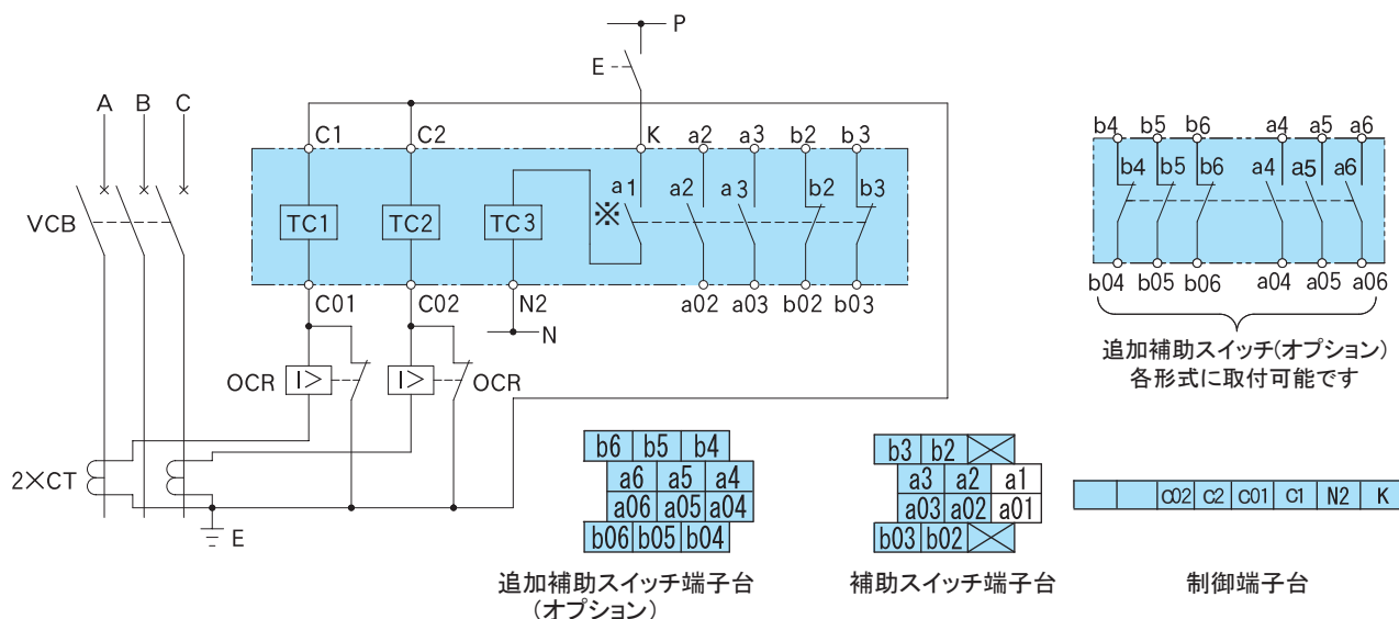
(d)CT二次電流引外し方式と電圧引外し方式
