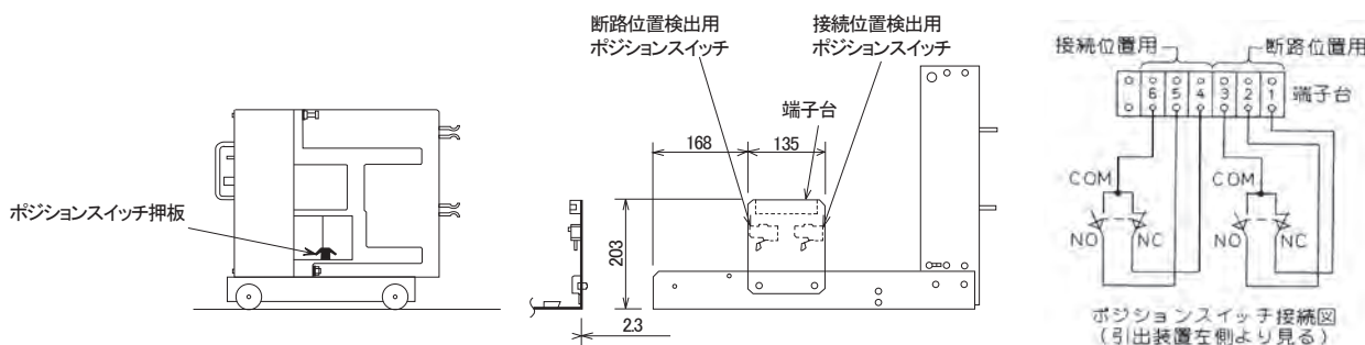
第23図 引出装置ポジションスイッチ部
