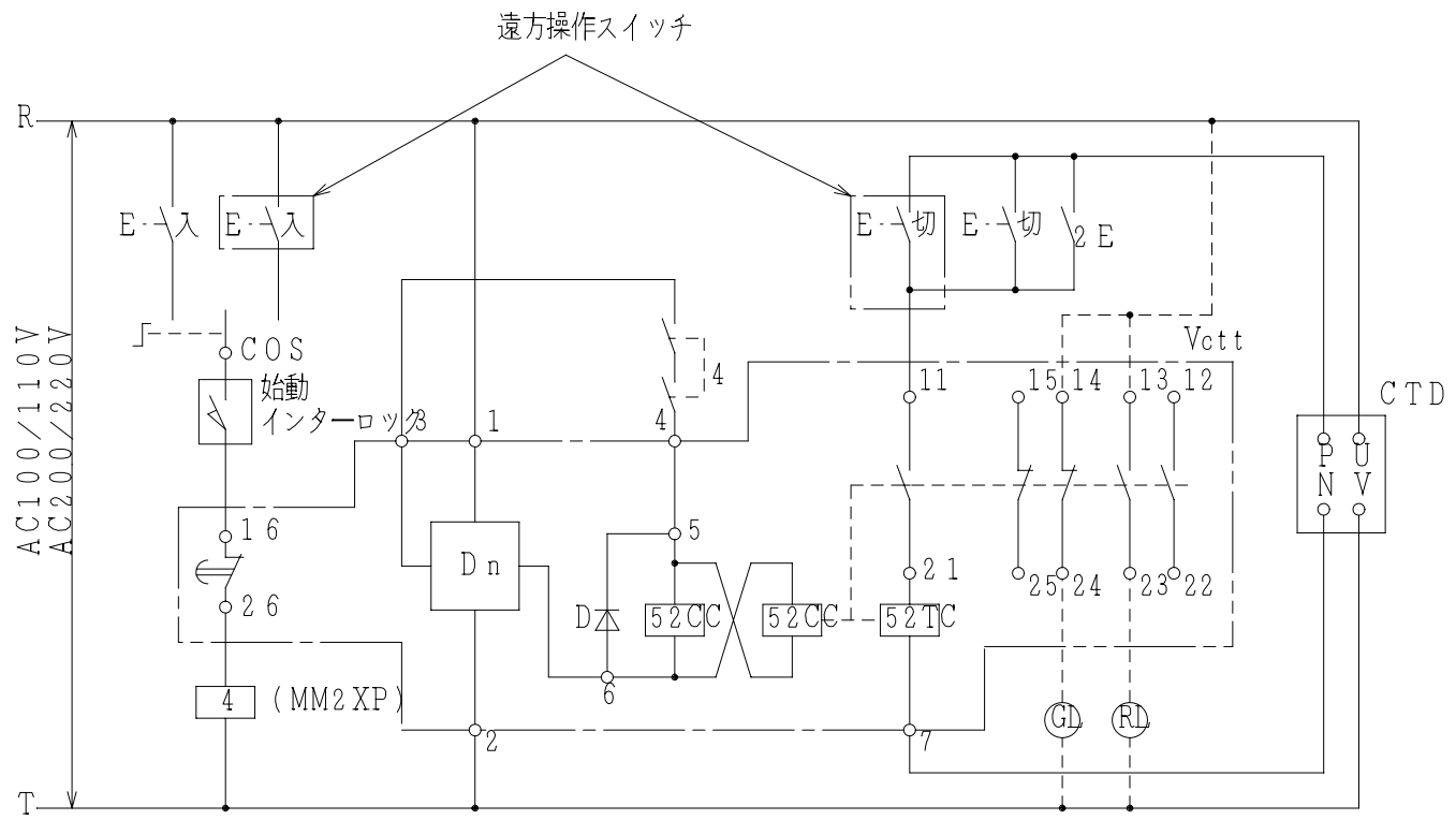
シヤントトリップ方式
