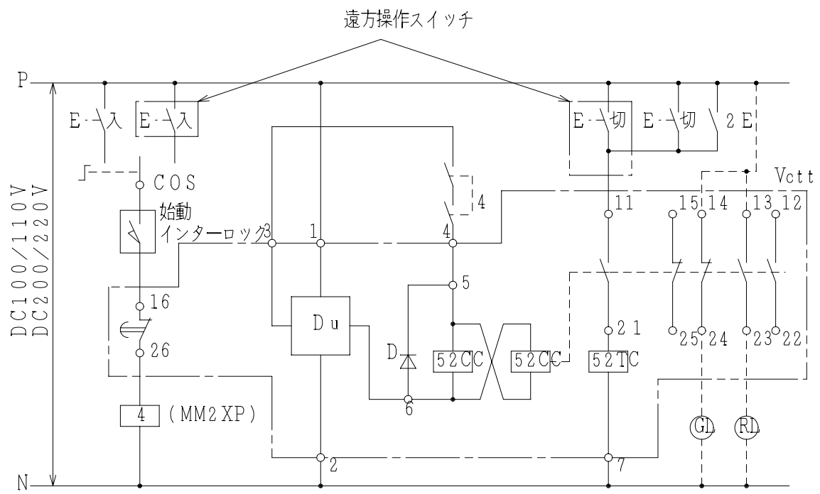
コンデンサトリップ方式
