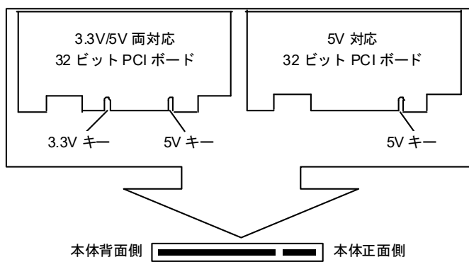
<スロット1~2のコネクタ形状>
