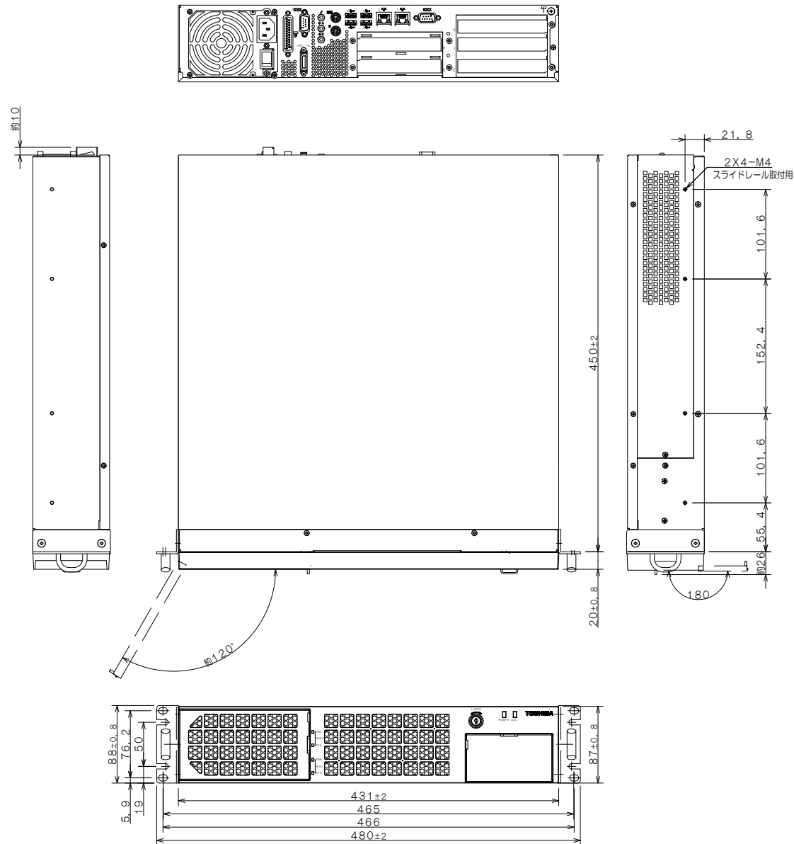
FR2100S model300/200外形図
