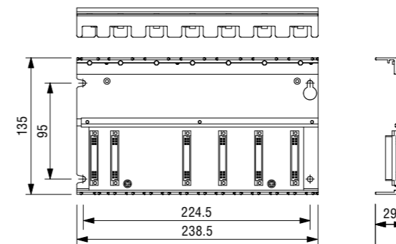
■ 基本/拡張ベースユニット(BU666) (単位:mm)
