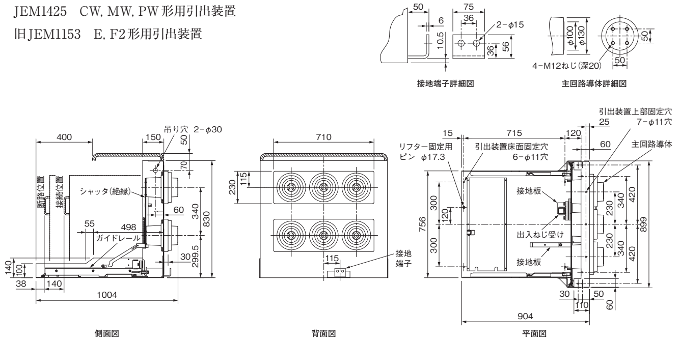
第 5 図 UKP-10QS引出装置外形寸法図
