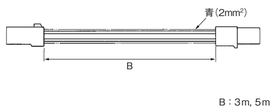
第16図 MIC コネクタ形用テストジャンパー線
