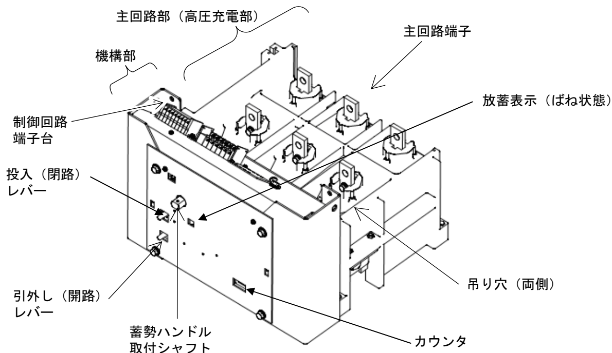
図3. 遮断器 MT形 (主回路端子上部前後)
