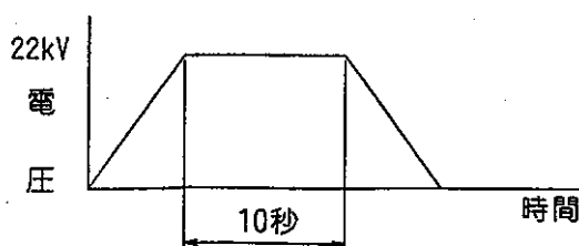
図 29. 電圧印加方法
