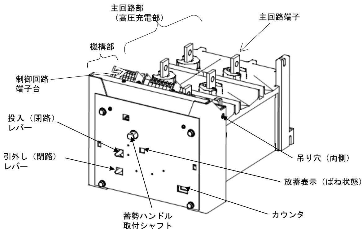
図 1. 遮断器 MU形 (主回路端子上下左右)
