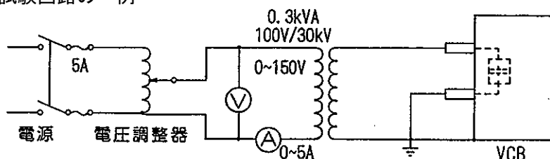
図 28. 耐電圧試験回路の一例
