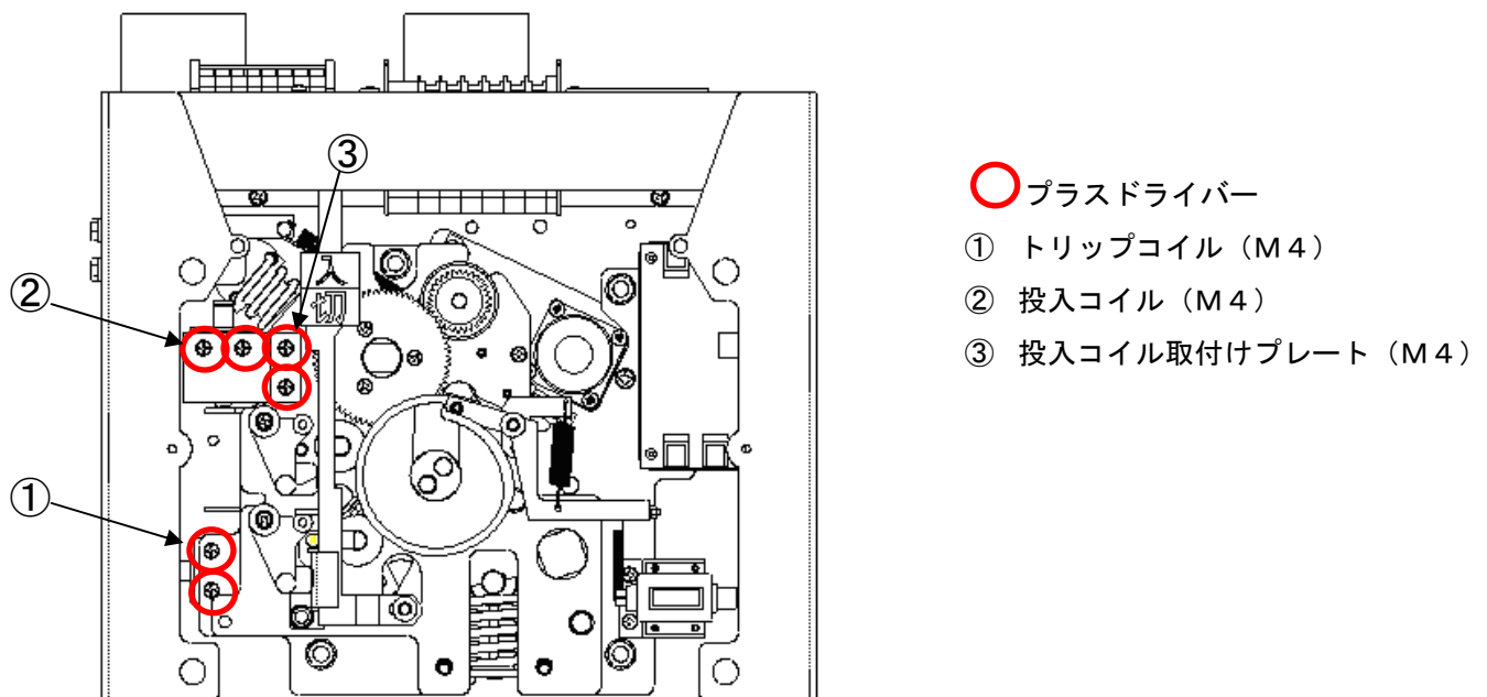
図 18. 操作機構部
