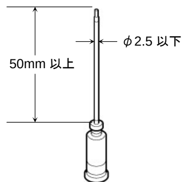
図 10. 推奨油差し
