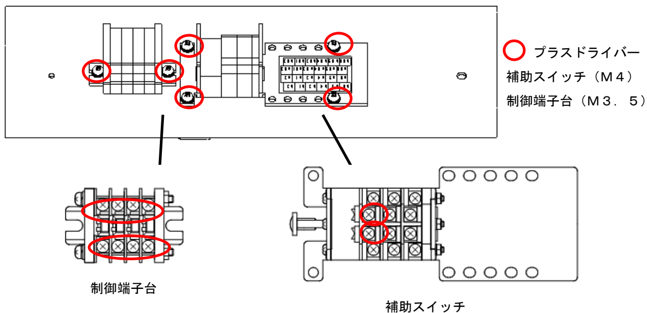
図 19. 制御回路部
