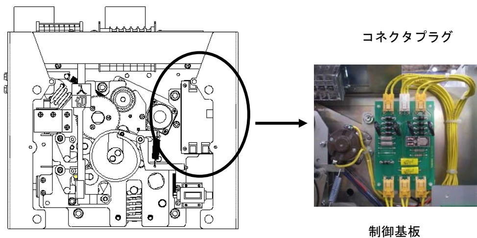
図 20. コネクタ接続確認
