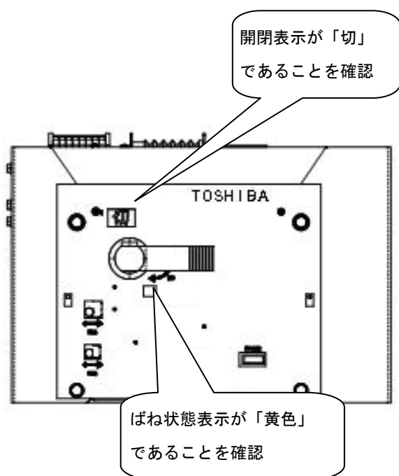
図23 遮断器の開閉状態表示が、「切」 ばね状態表示が、「黄色」 であることを確認する。
