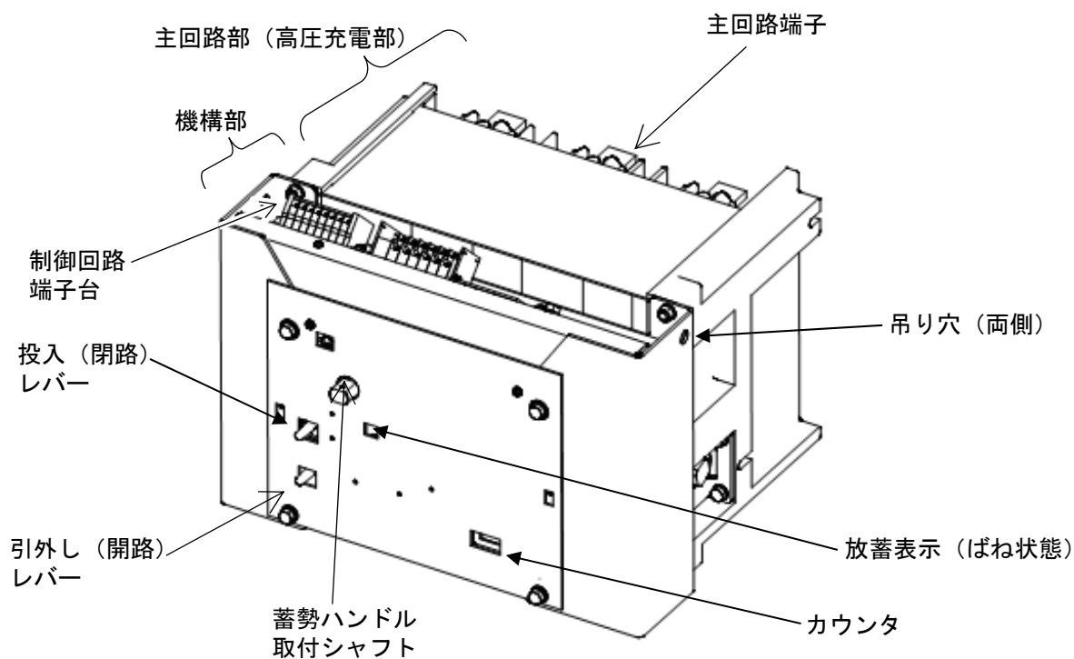
図 2. 遮断器 ML形 (主回路端子背面水平)
