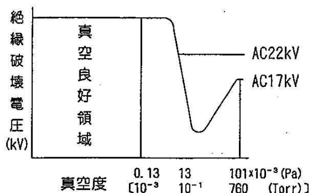
図 27. 絶縁破壊特性
