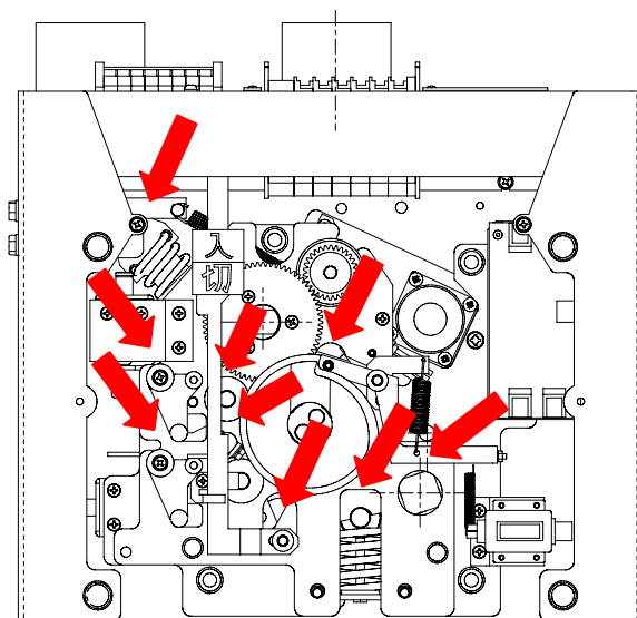
図 1 4 操作機構部
