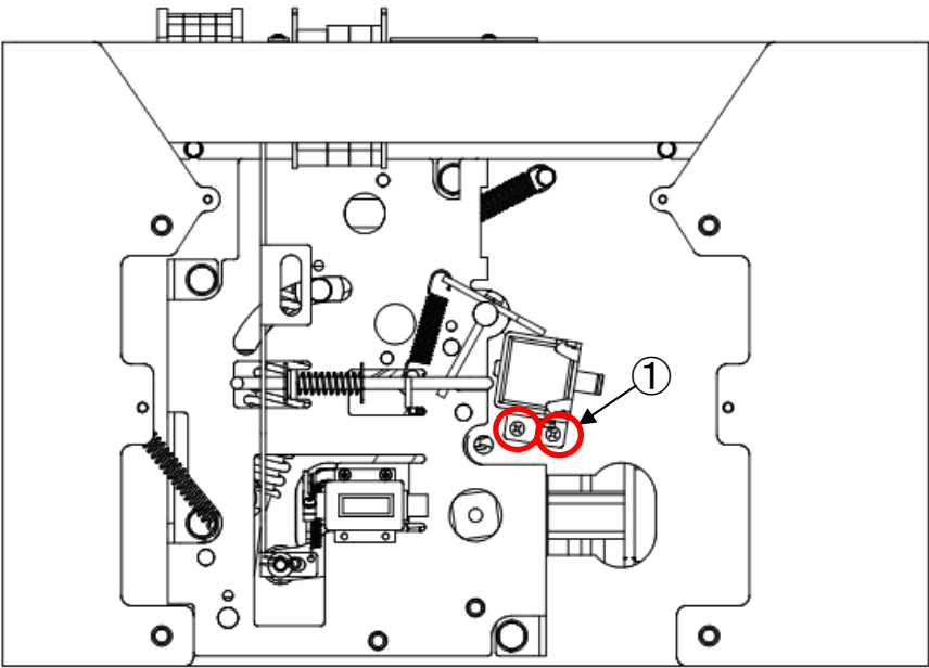
図 14. 操作機構部
