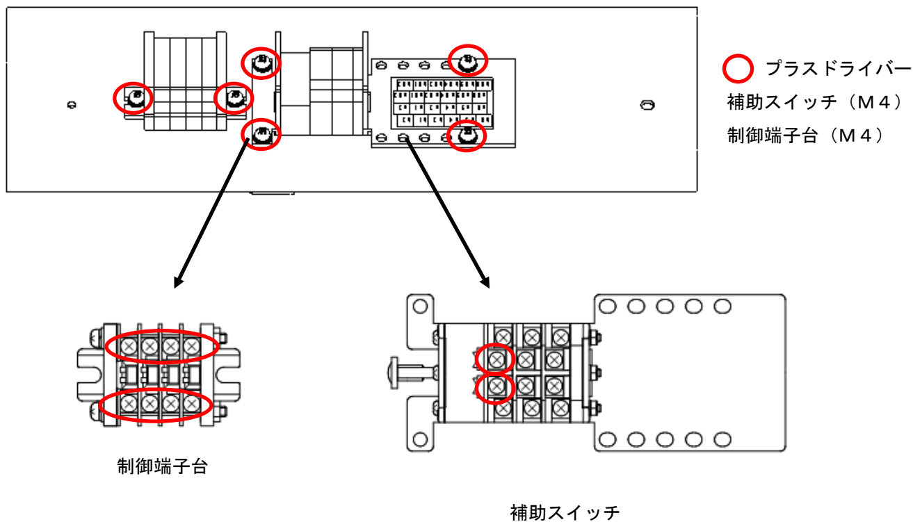
図 1 5 . 制御回路部
