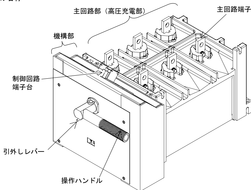
図 1. U 形（主回路端子上部左右）
