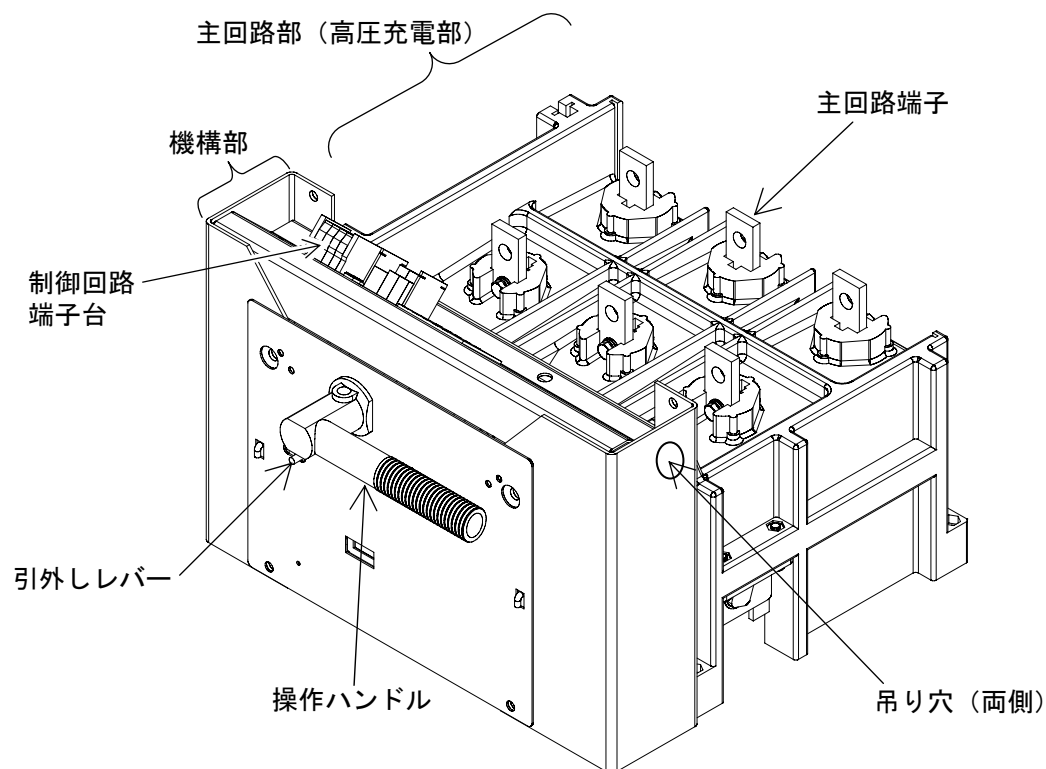
図3. T形（主回路端子上部前後）
