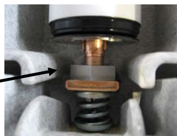
図7 清掃箇所（シャフト部）
