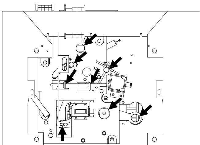
図 1 2 操作機構部
