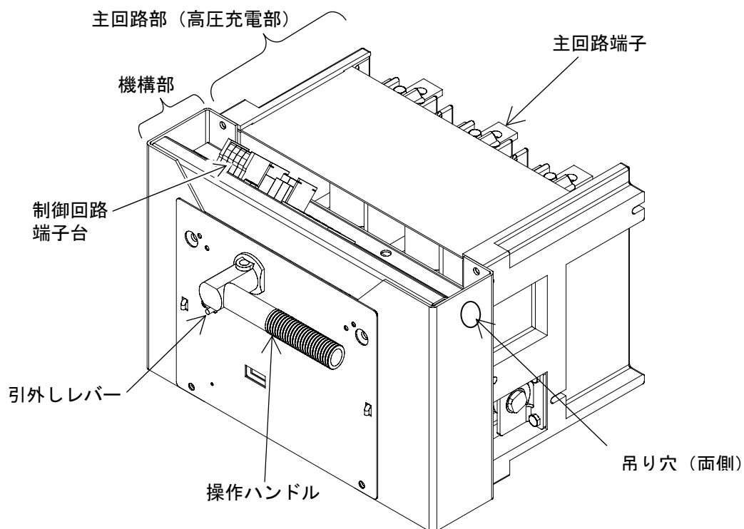
図 2. L 形（主回路端子背面水平）
