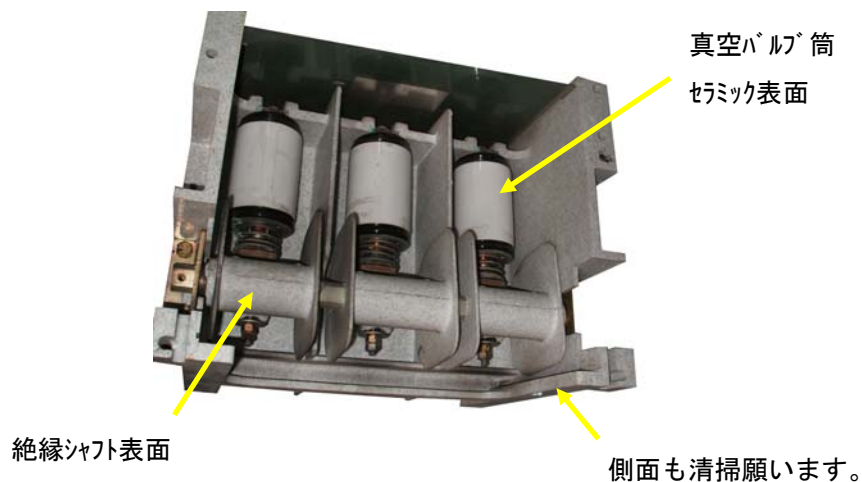
図 6. 清掃箇所
