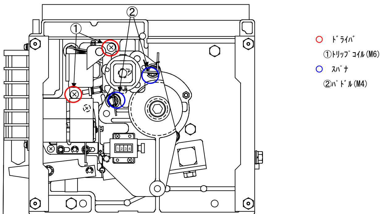
図 11. ねじ締付確認
