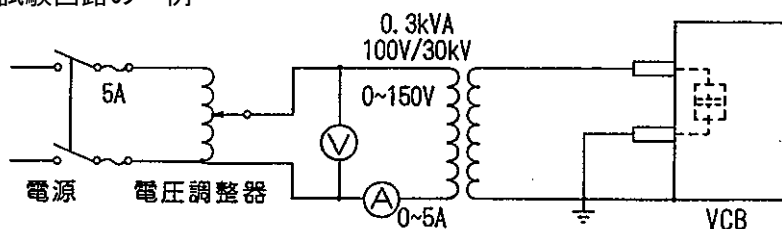
図 15. 耐電圧試験回路の一例
