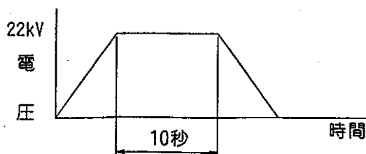
図 16. 電圧印加方法
