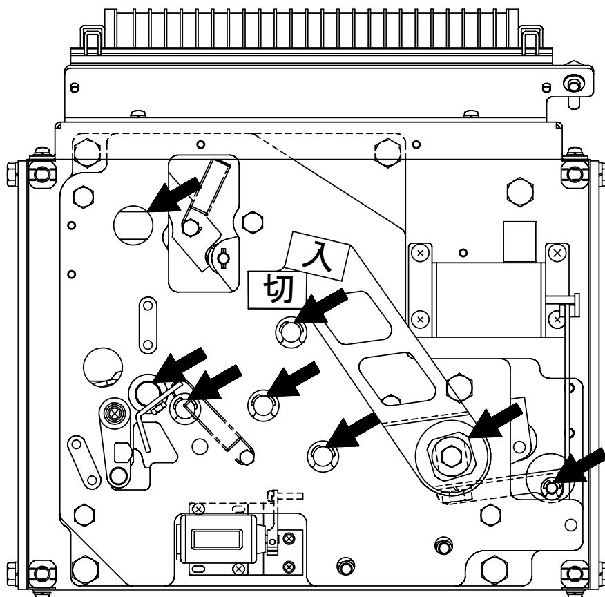
図 9. 操作機構部正面図 (全機種共通)
