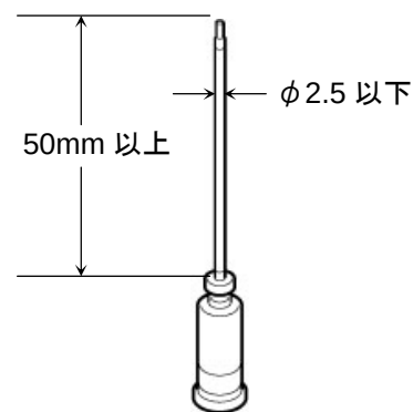
図8. 推奨油差し
