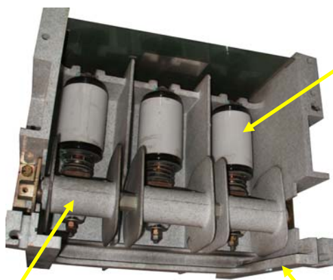
真空バルブ筒 セラミック表面
