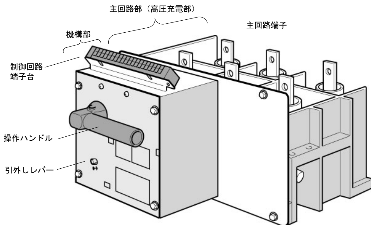
図 3. T 形（主回路端子上部前後）
