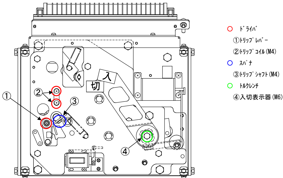
図 11. 操作機構部
