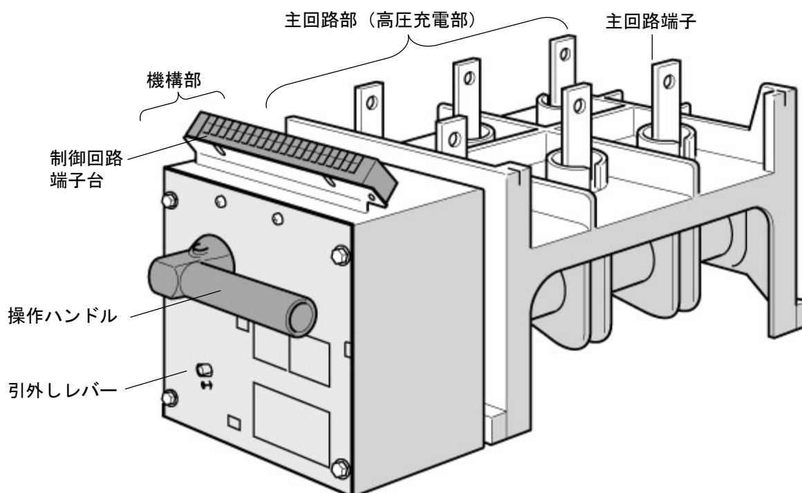
図 1. U 形（主回路端子上部左右）
