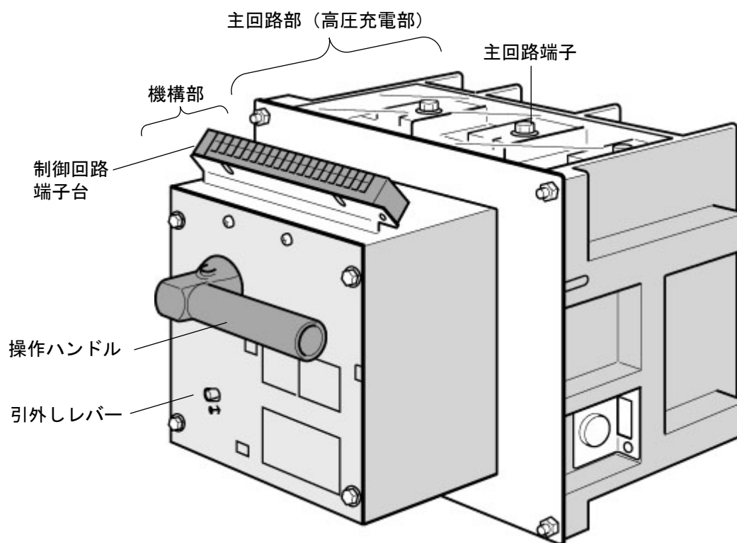
図 2. L 形（主回路端子背面水平）
