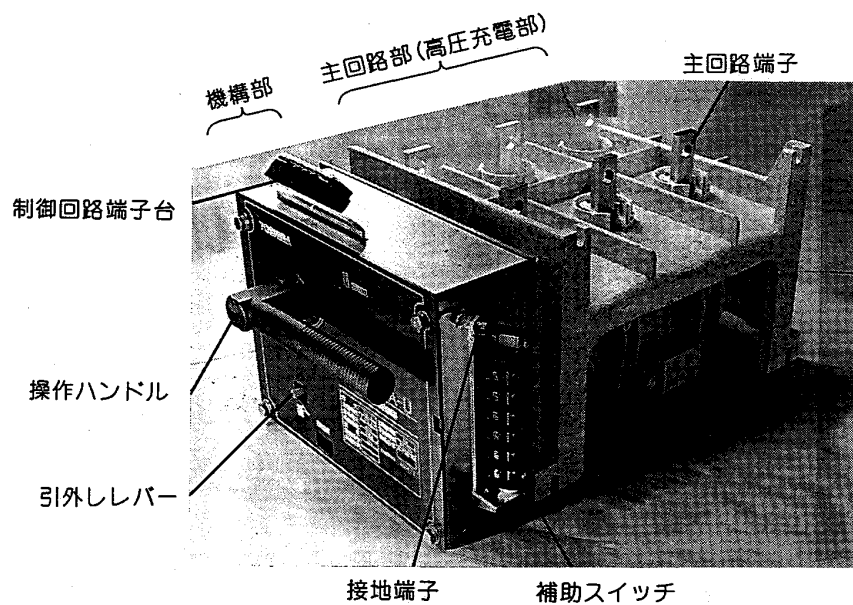
図 1. U 形 (主回路端子上部左右)
