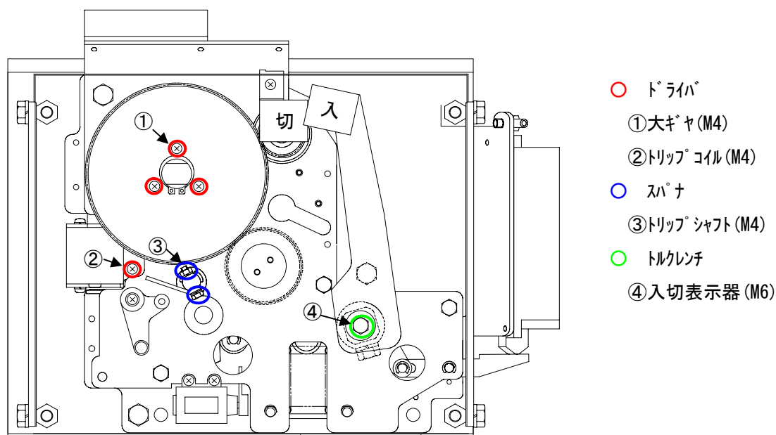
図 11. 操作機構部
