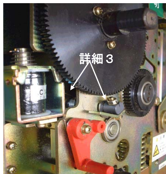
図 9. 給油・注油箇所図 1
