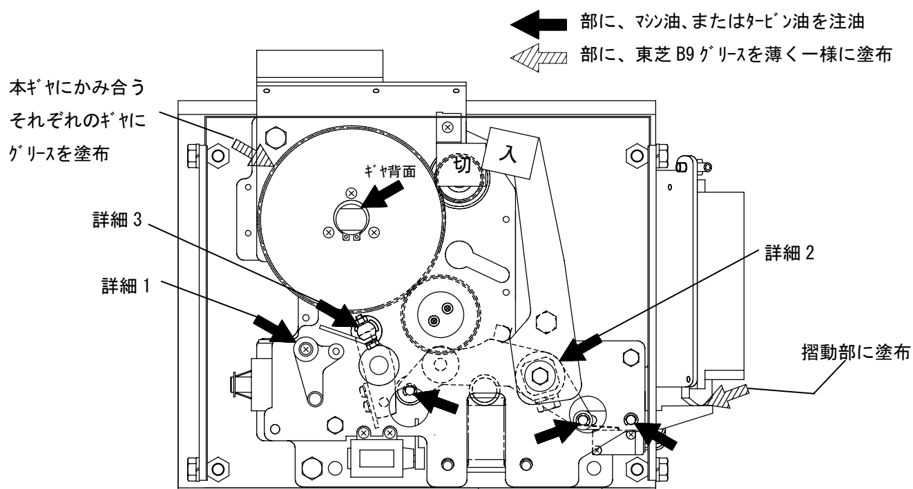
操作機構部正面図
