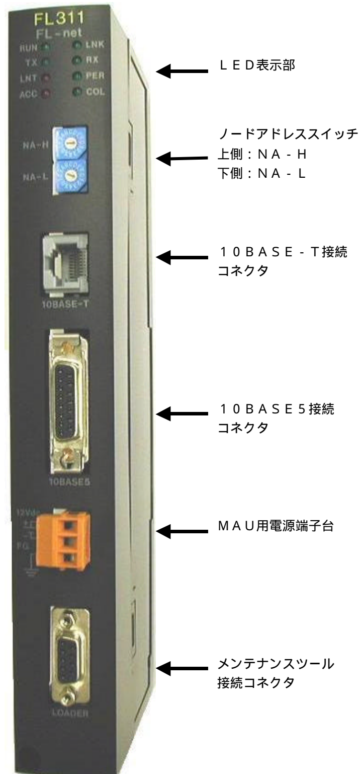
図 3.1 FL311の各部位
