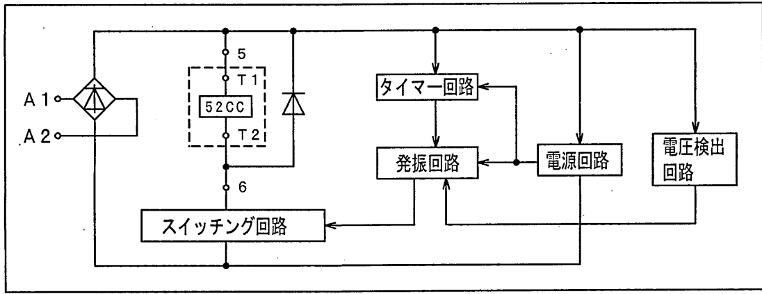
ドライブユニット構成図
