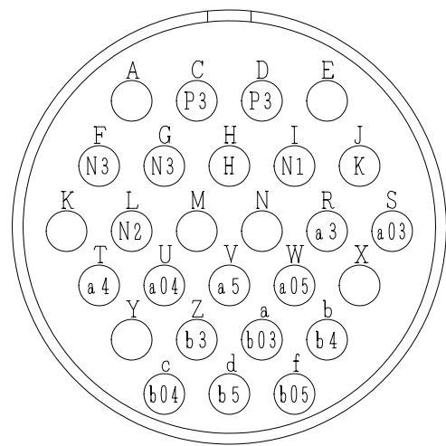
接続プラグ ( 1 )
