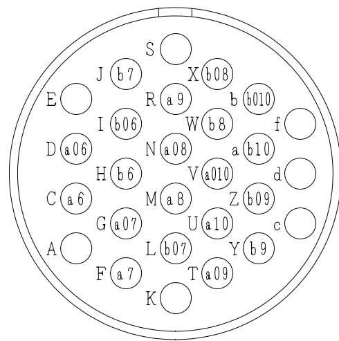
接続プラグ ( 2 )
