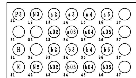
制御回路断路部詳細図(遮断器正面より)
