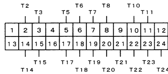
制御回路コネクタ
