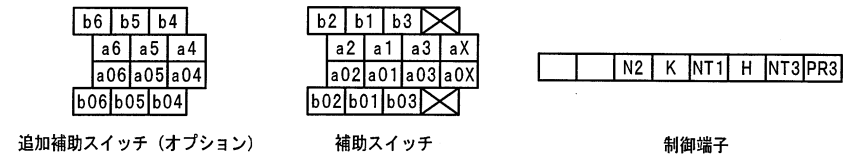
端子配列図 (真空遮断器背面より見る)
