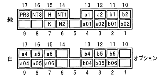
制御回路断路部配置図
