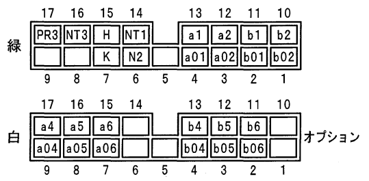
制御回路断路部配置図
