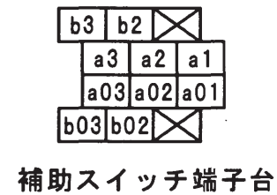
端子配列図（真空遮断器背面より見る）
