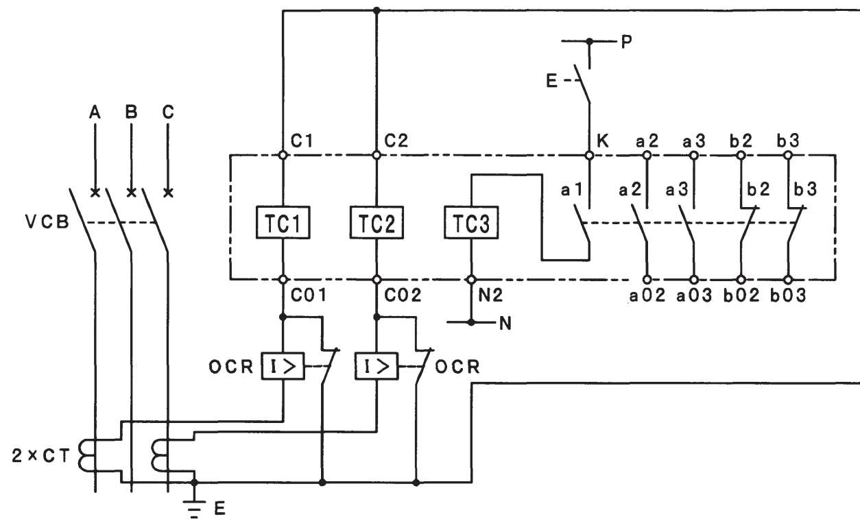
電流引外し方式（電圧引外しコイル付）
