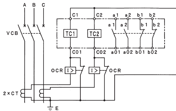
電流引外し方式
