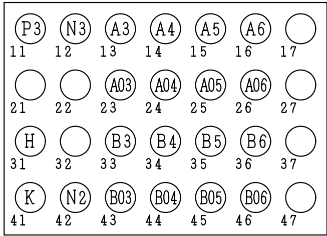
制御回路断路部配置図
