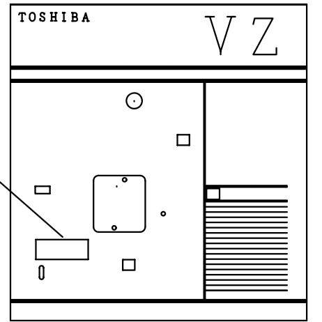
制御回路断路部配置図
