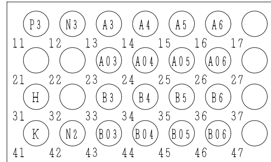
制御回路断路部配置図 (遮断器正面より)
