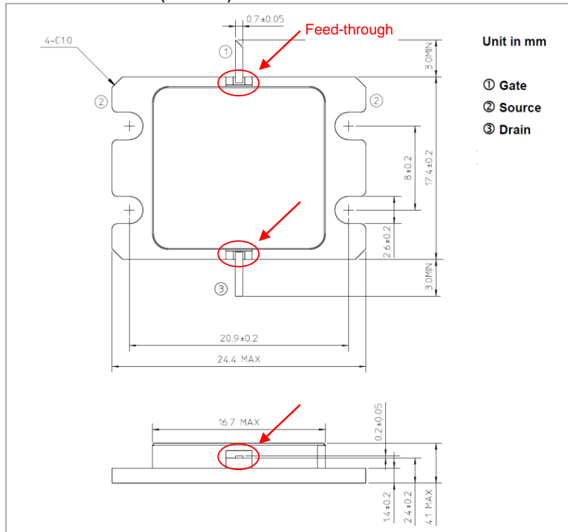
PACKAGE OUTLINE (7-AA06A)
