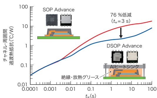
(a) 過渡熱抵抗の比較
