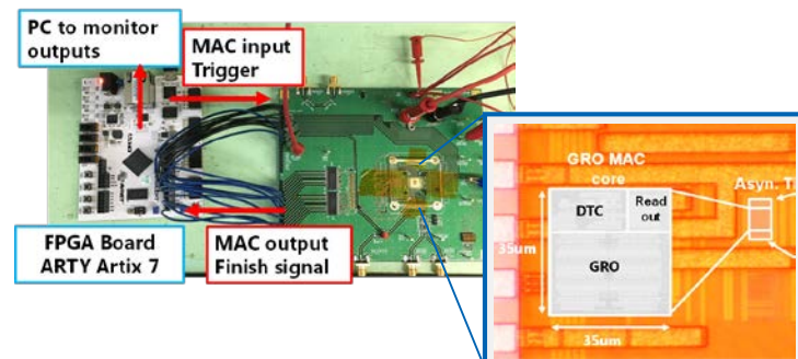
評価ボード・試作チップ(28nmCMOS技術)
