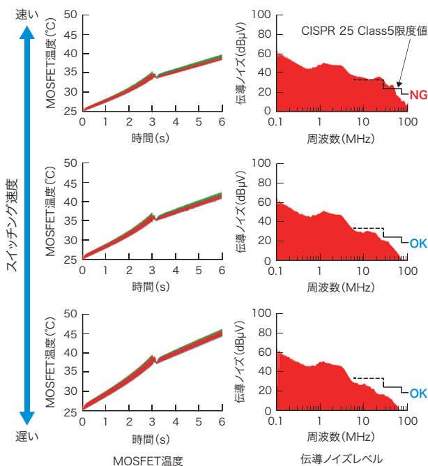
図5. スwitchング速度を変えたときの発熱とノイズの検証結果
