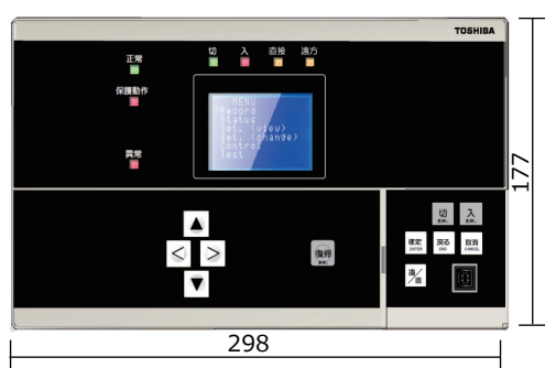
前面図
