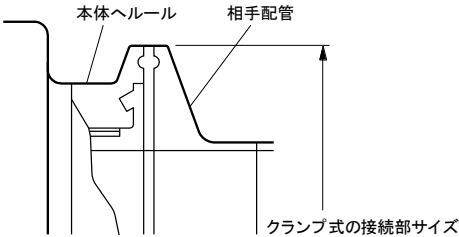
図 11 相手配管と接続する部分の位置
