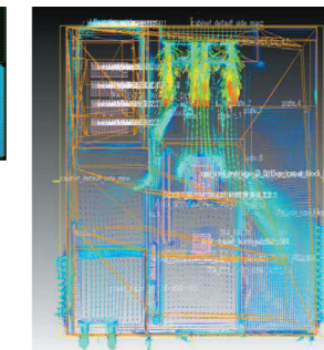
熱流体解析
