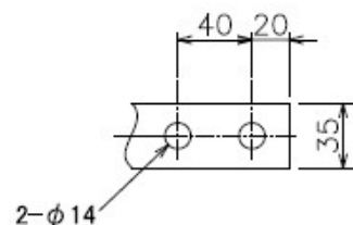
主回路導体詳細図
