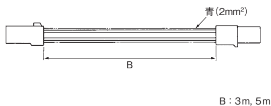
第16図 MIC コネクタ形用テストジャンパー線
