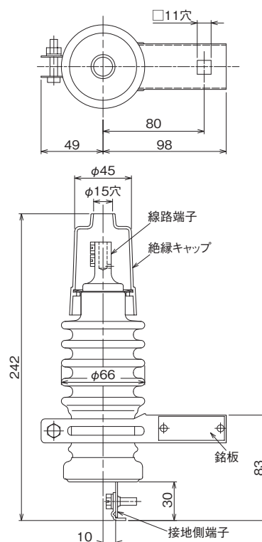
第24図 RVSQ-3GPS, 6GPS (L2) 形避雷器外形寸法図
