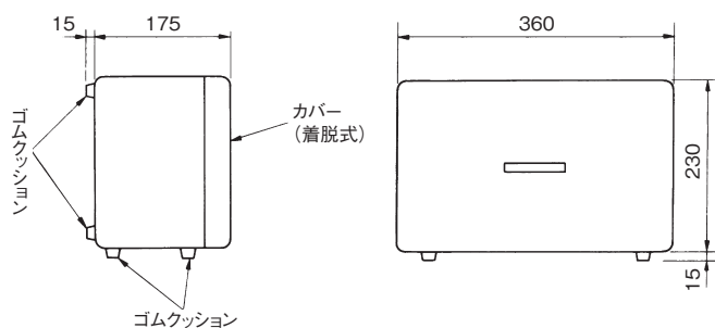
第26図 CI35-1D耐電圧チェッカ外形寸法図
