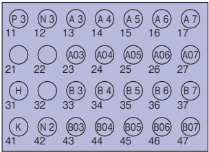
制御回路断断路部配置図 (遮断器正面より) (プラグインロック用コネクタの場合)
