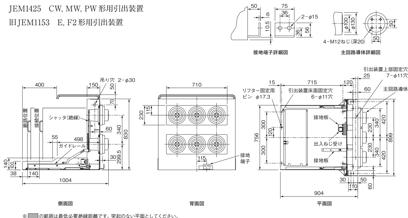
第 5 图 UKP-10QS引出装置外形寸法图
