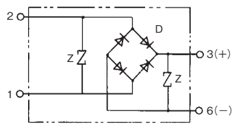
内部接続図
