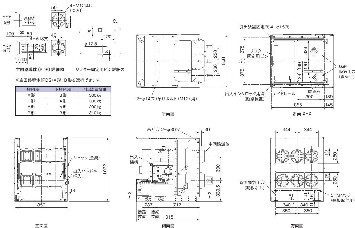
第 6 图 UZP-6RS 引出装置外形寸法图
