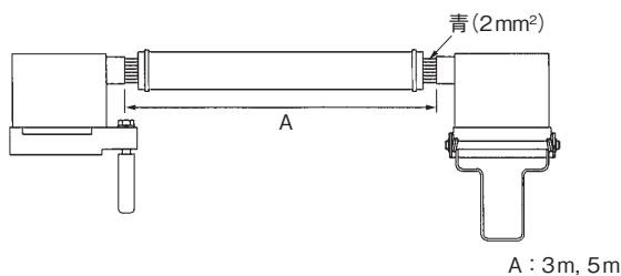
第15図 プラグインタロック形用テストジャンパー線
