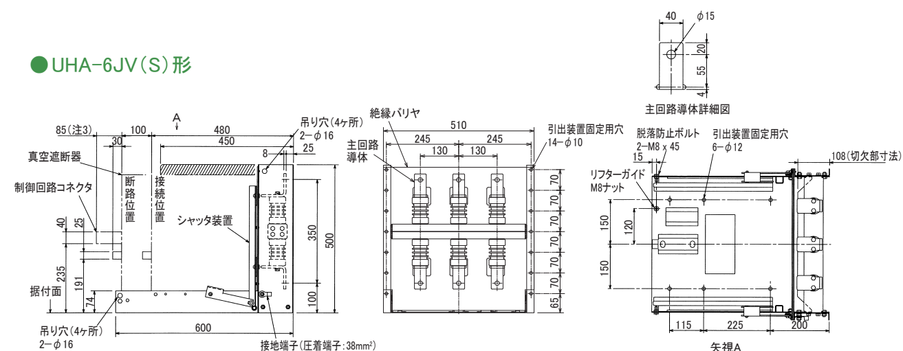
第 18 图 UHA-6JV(S)形引出装置外形寸法图
