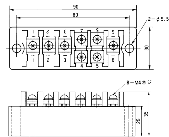
(外形寸法図)
