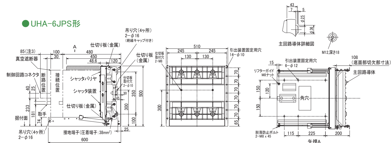
第 19 图 UHA-6JPS 形引出装置外形寸法图
