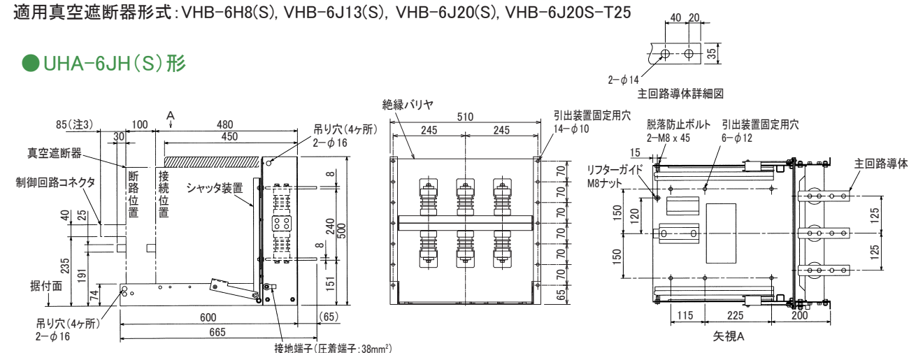
第 17 图 UHA-6JH(S)形引出装置外形寸法图
