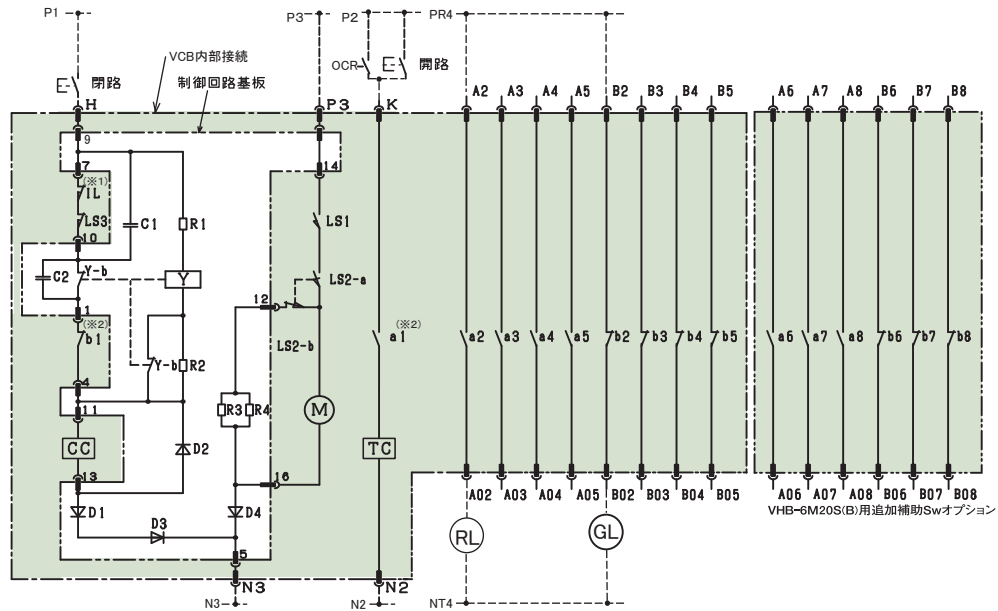
直流投入、引外し操作接続図
