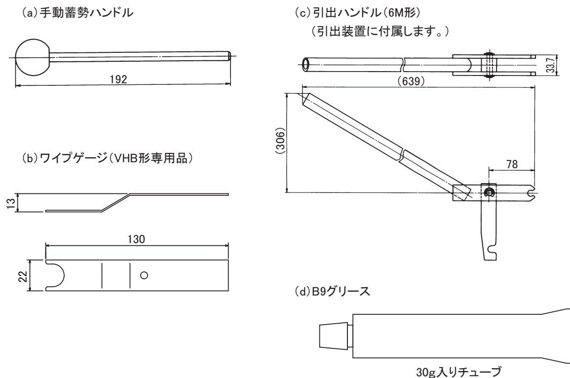
第 26 図 標準付属品
