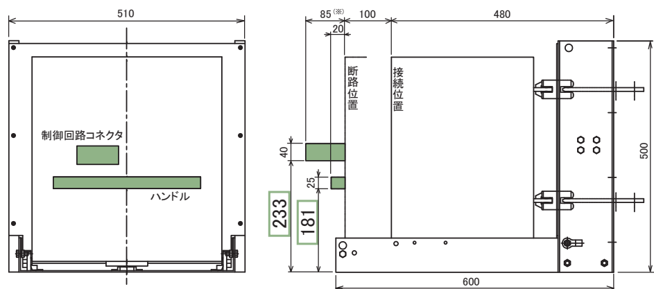
第 45 図 VH-6J13S(VH-6H8S,VH-6J20S)、VHA-6J13S(VHA-6H8S,VHA-6J20S)の引出装置収納状態
