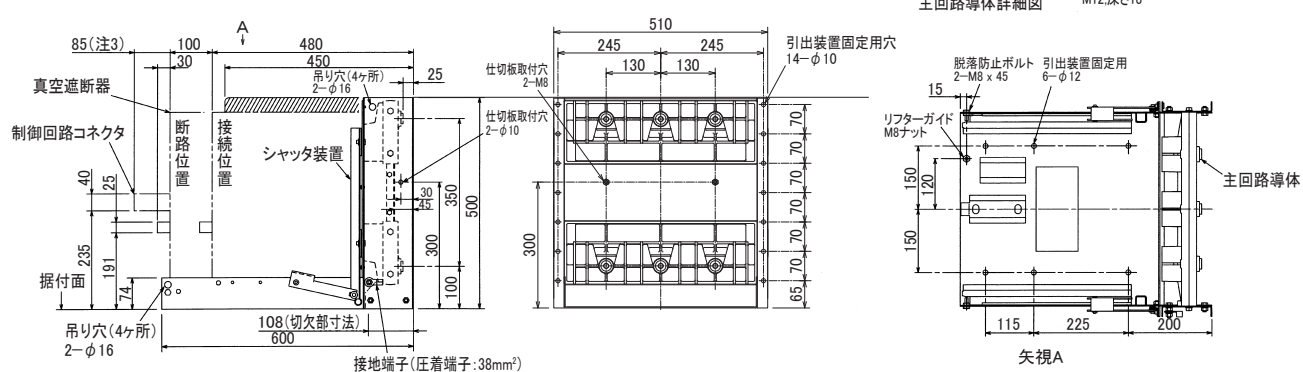
第19図 UHA-6JPS形引出装置外形寸法図
