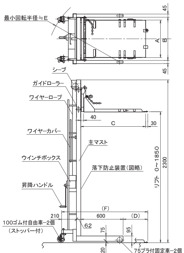
第 35 図 リフター
