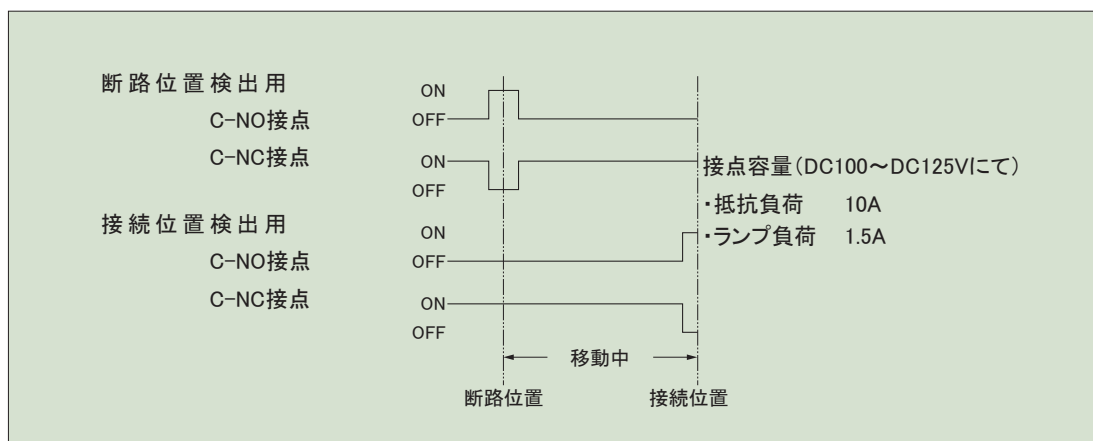
第 25 図 接点動作タイミング
