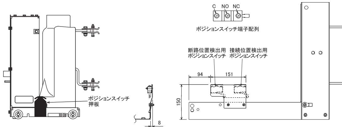
第 23 図 ポジションスイッチ (UHA-6J)
