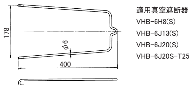
第 32 図 吊り金具
