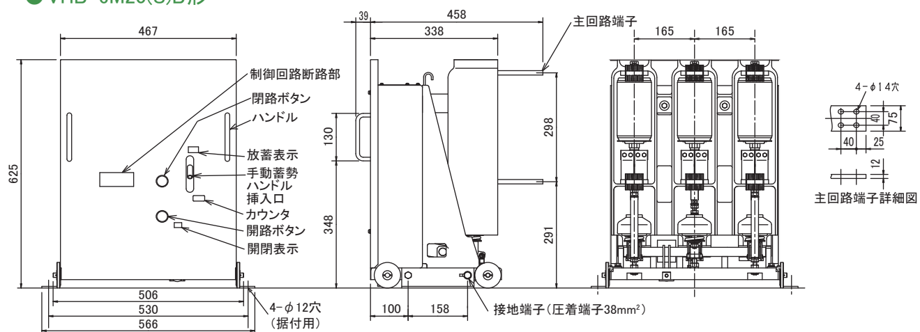
第 13 図 VHB-6M20(S)B 固定形真空遮断器外形寸法図
