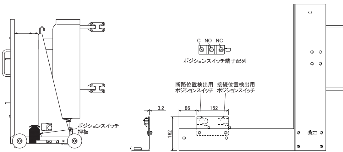
第 24 図 ポジションスイッチ (UHA-6M)
