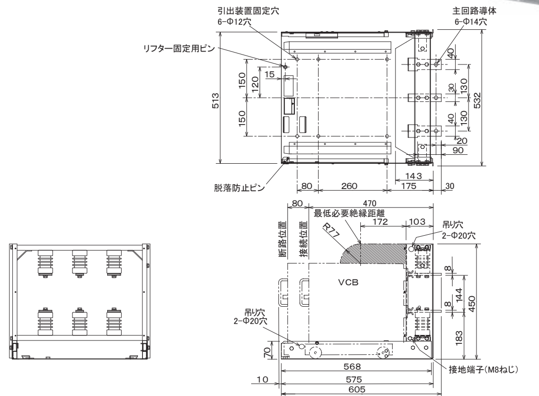
第10図 U6A-HL1形水平引出装置外形寸法図(導体方向水平)
