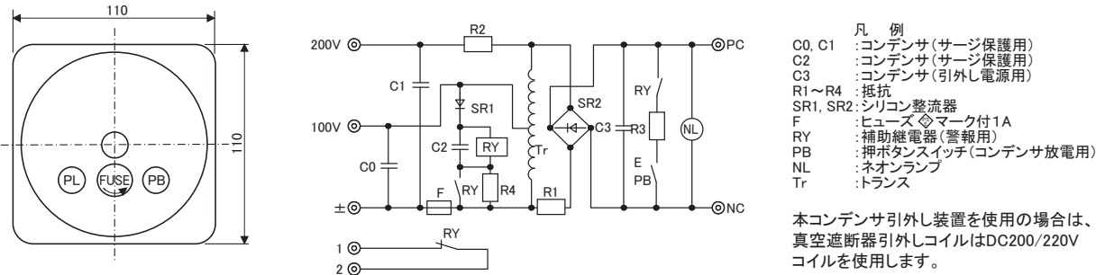
第30図 コンデンサ引外し装置CIT-10Q
