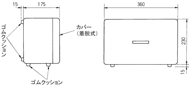
(b) 耐電圧チェッカ寸法
