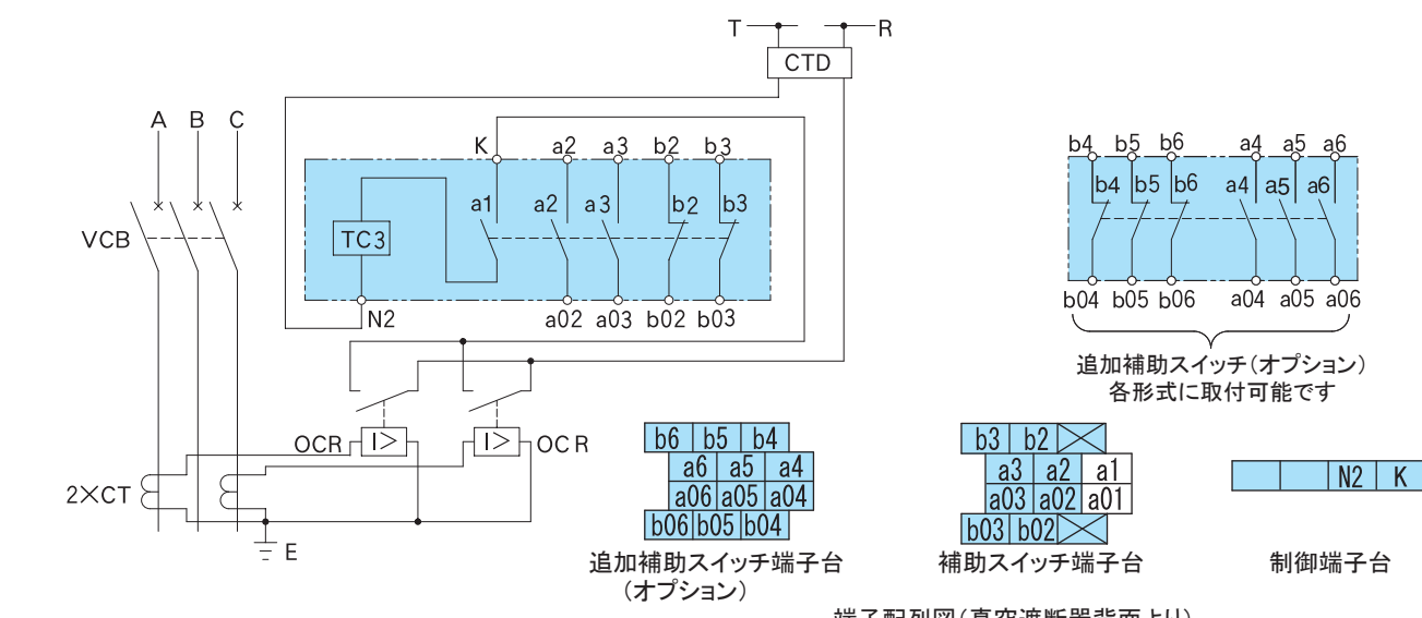
(c) コンデンサ引外し方式
