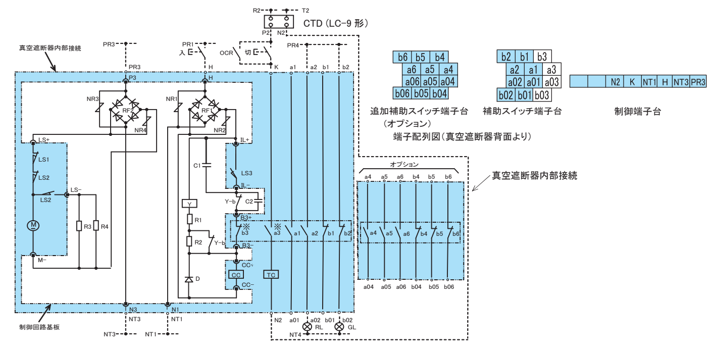
(b) コンデンサ引外し方式
