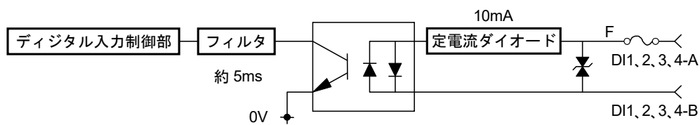
参考接続例
