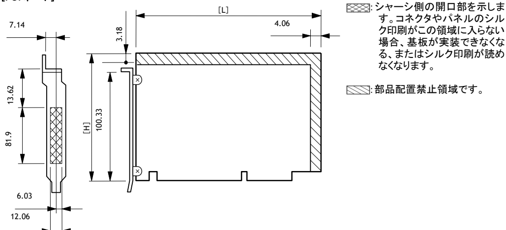
【PCI ボード】
