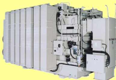
油入変圧器 ~50MVA
